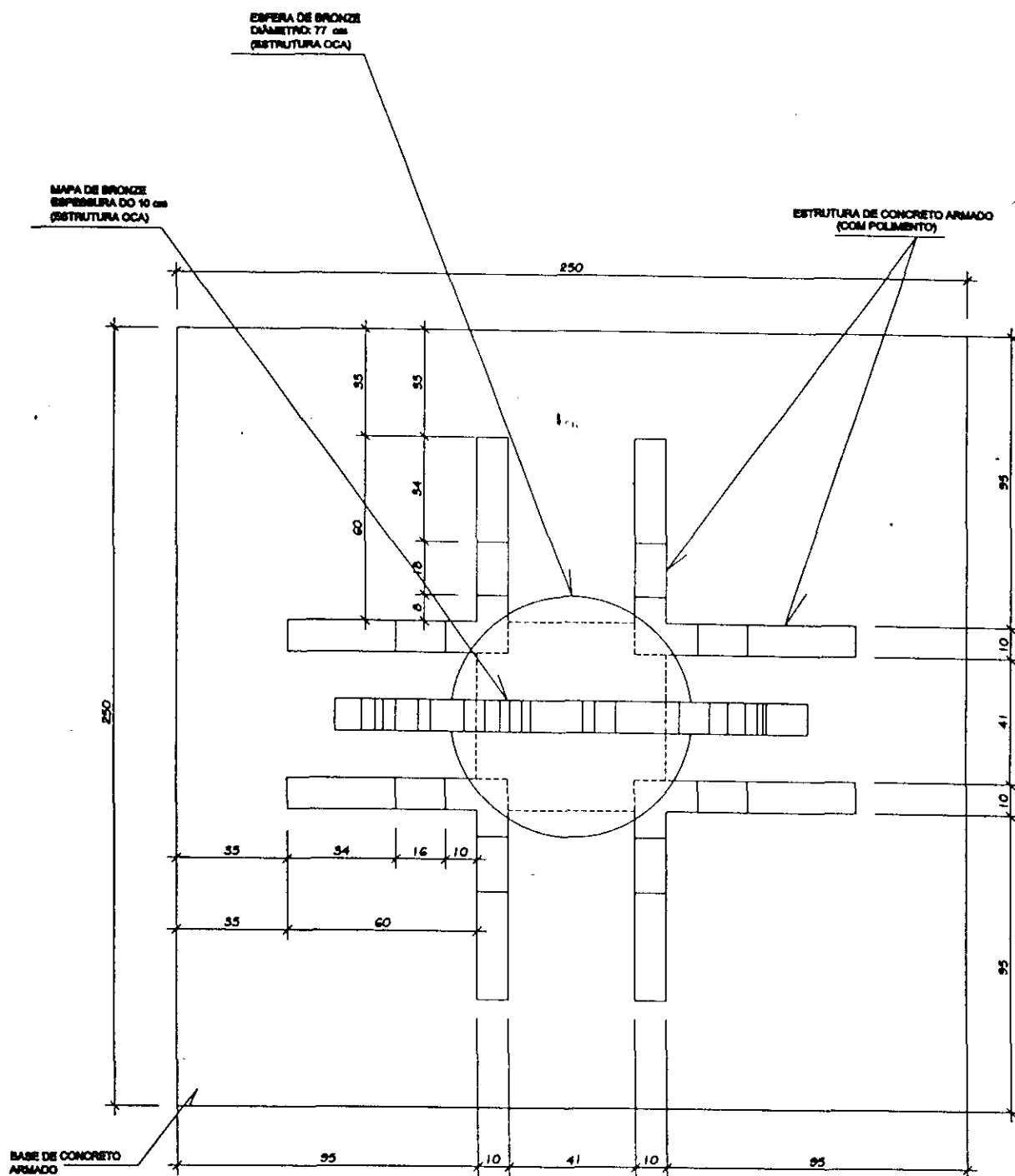
VISTA SUPERIOR S/ESCALA MONUMENTO: PRAÇA TIRADENTES
