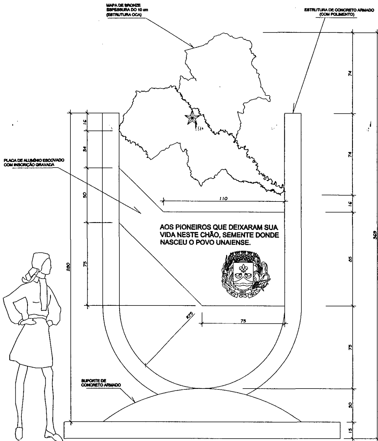
VISTA FRONTAL S/ESCALA MONUMENTO: PRAÇA TIRADENTES
