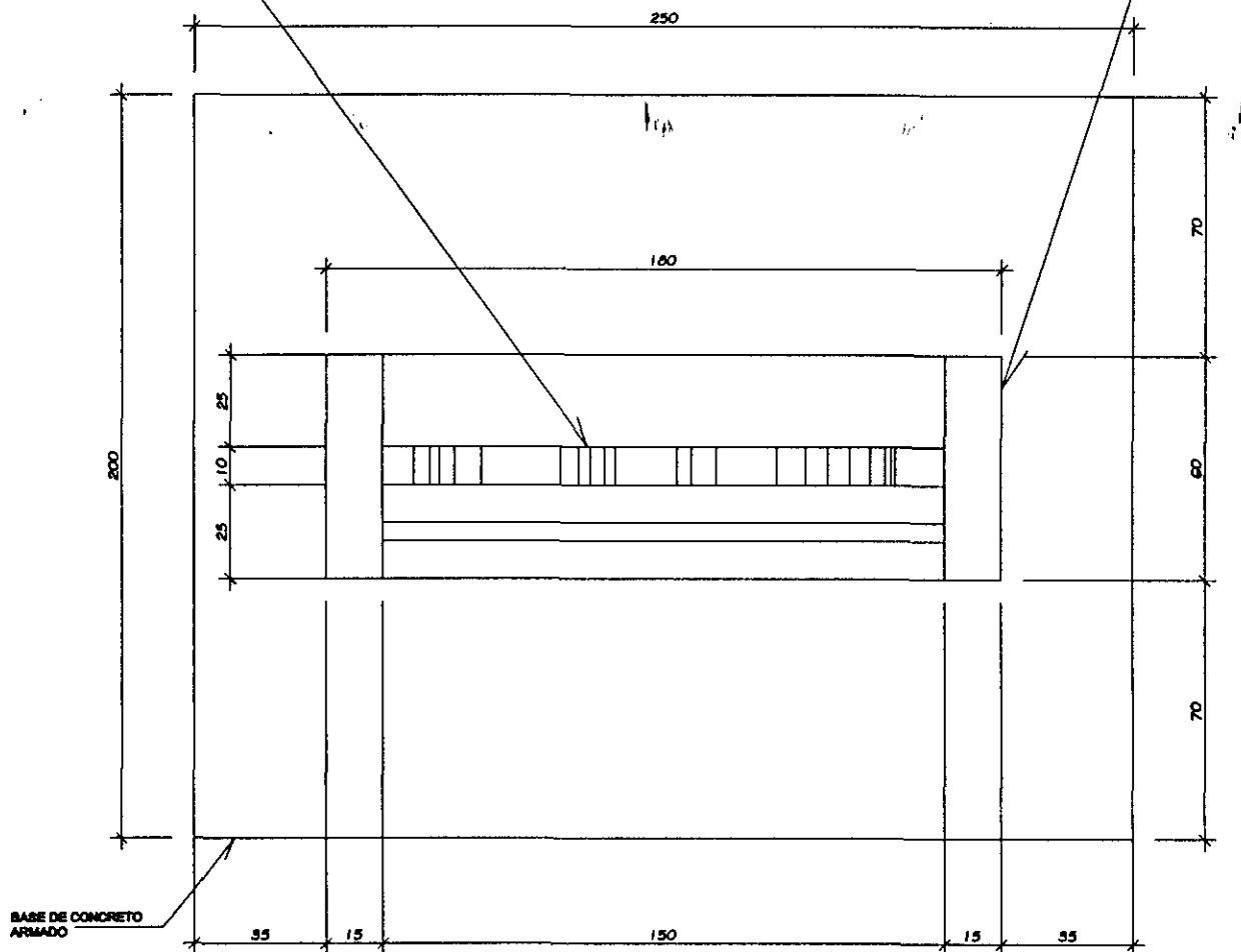
VISTA SUPERIOR S/ESCALA MONUMENTO: PRAÇA TIRADENTES
